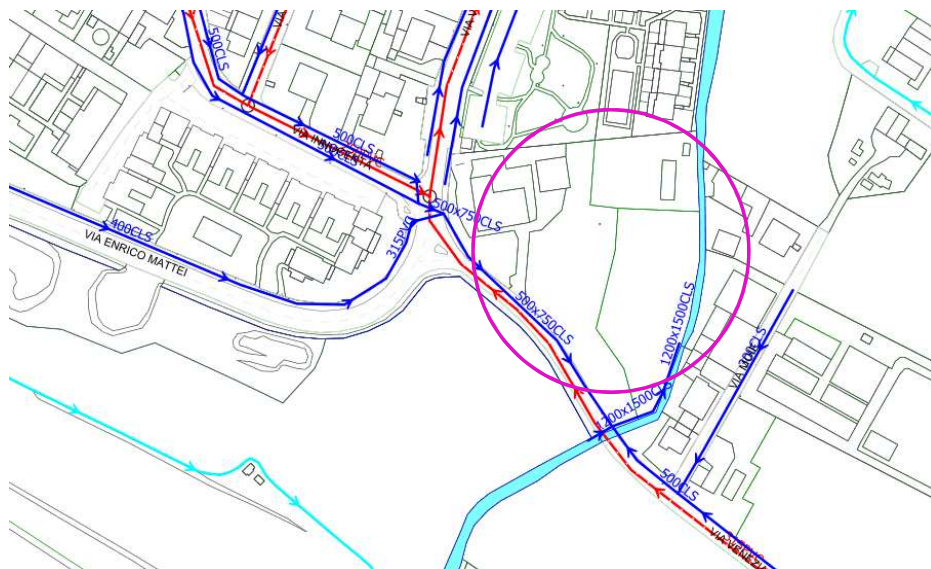
PL.01- Planimetria rete fognaria comunale.
