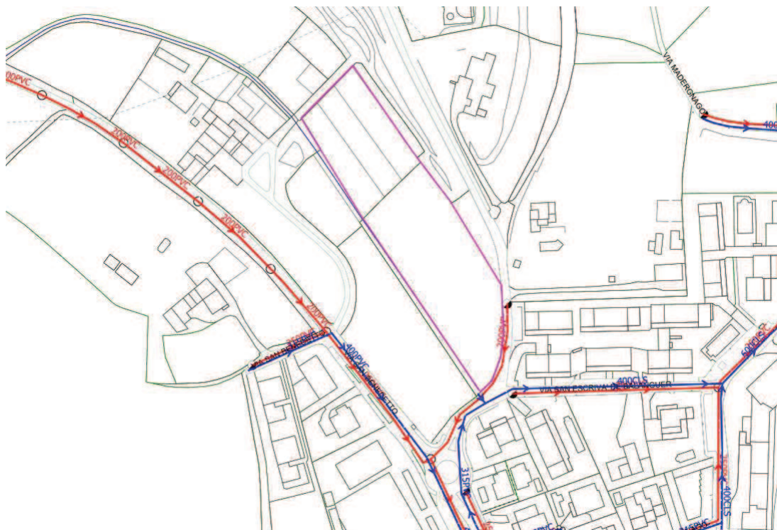
PL.01- Planimetria rete fognaria comunale.
