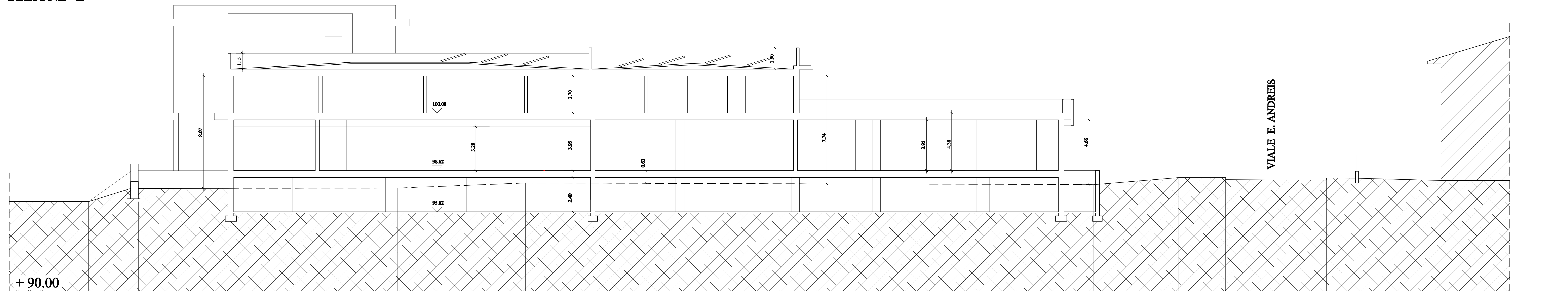
SEZIONE 3
