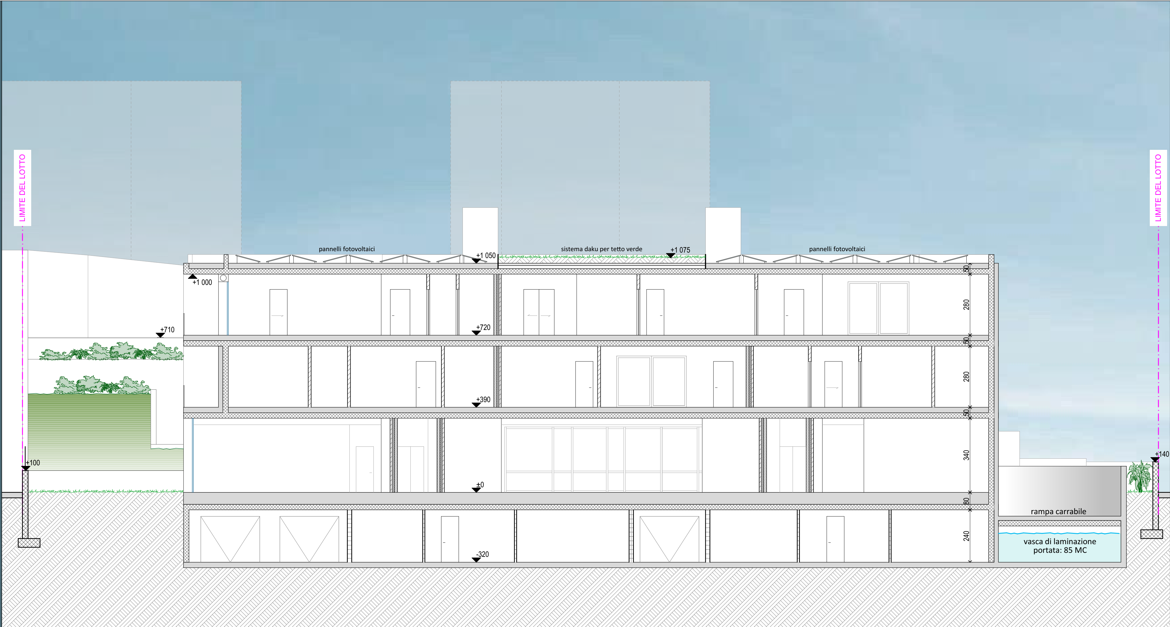
SEZIONE A-A
