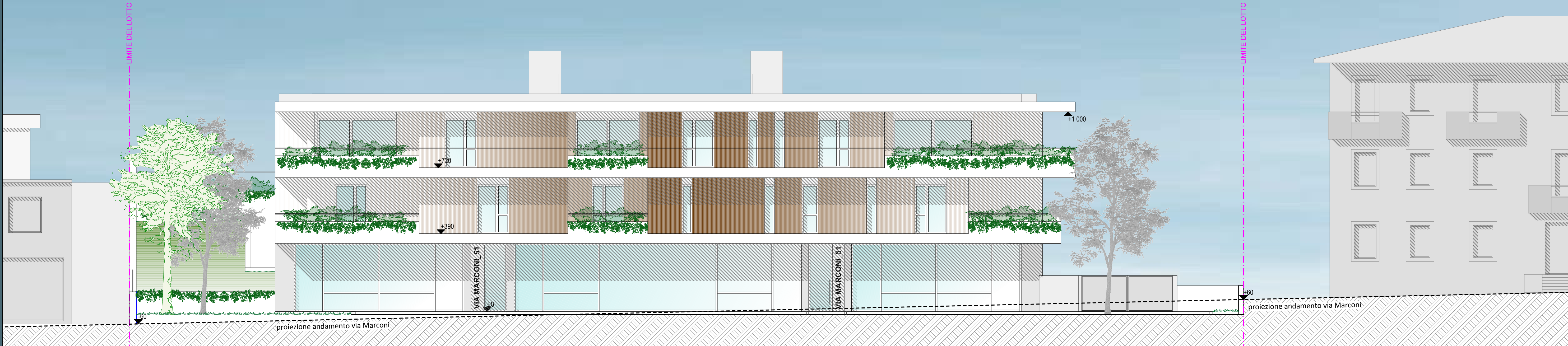
PROSPETTO NORD FRONTE VIA MARCONI
