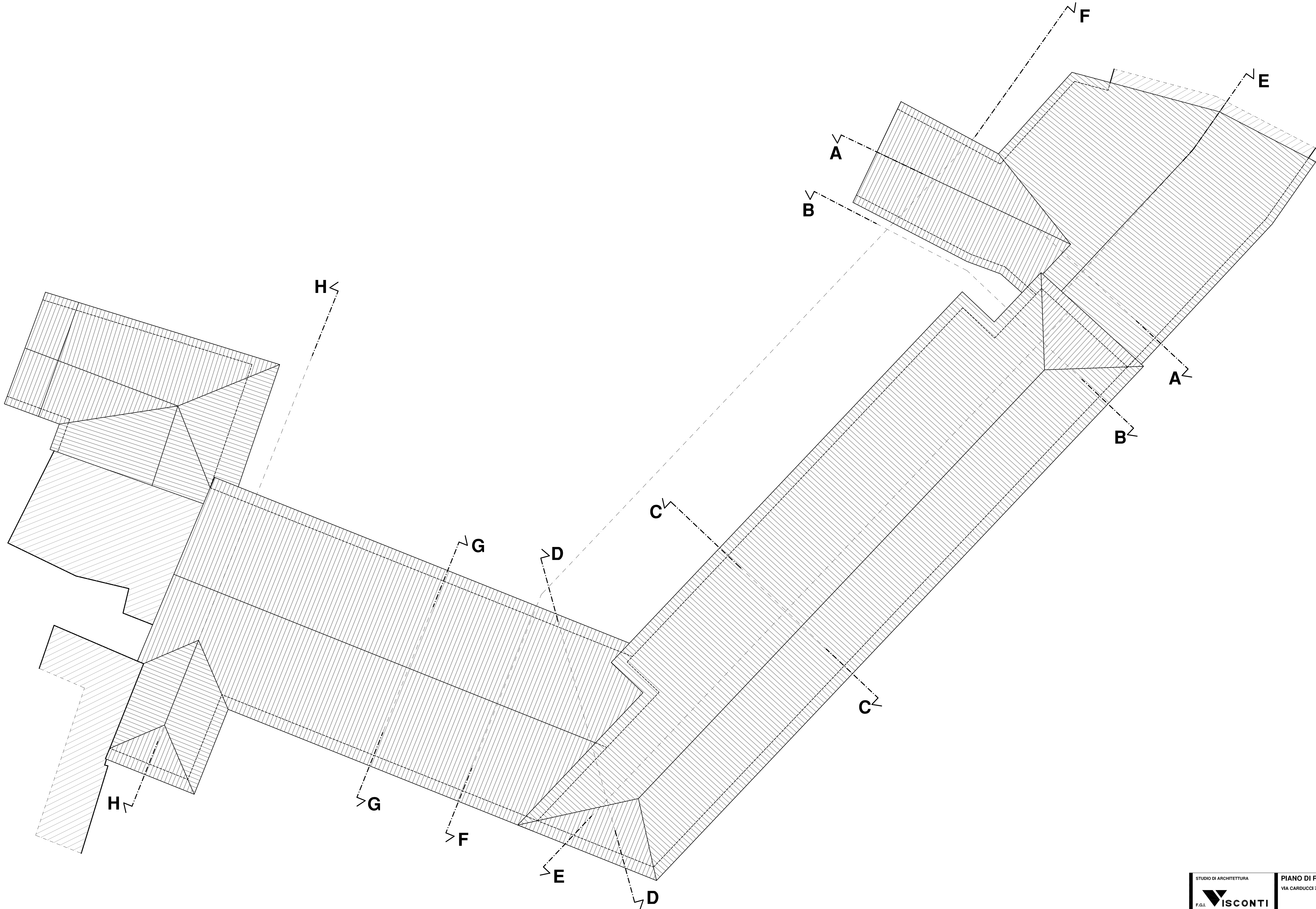
PIANO COPERTURA
