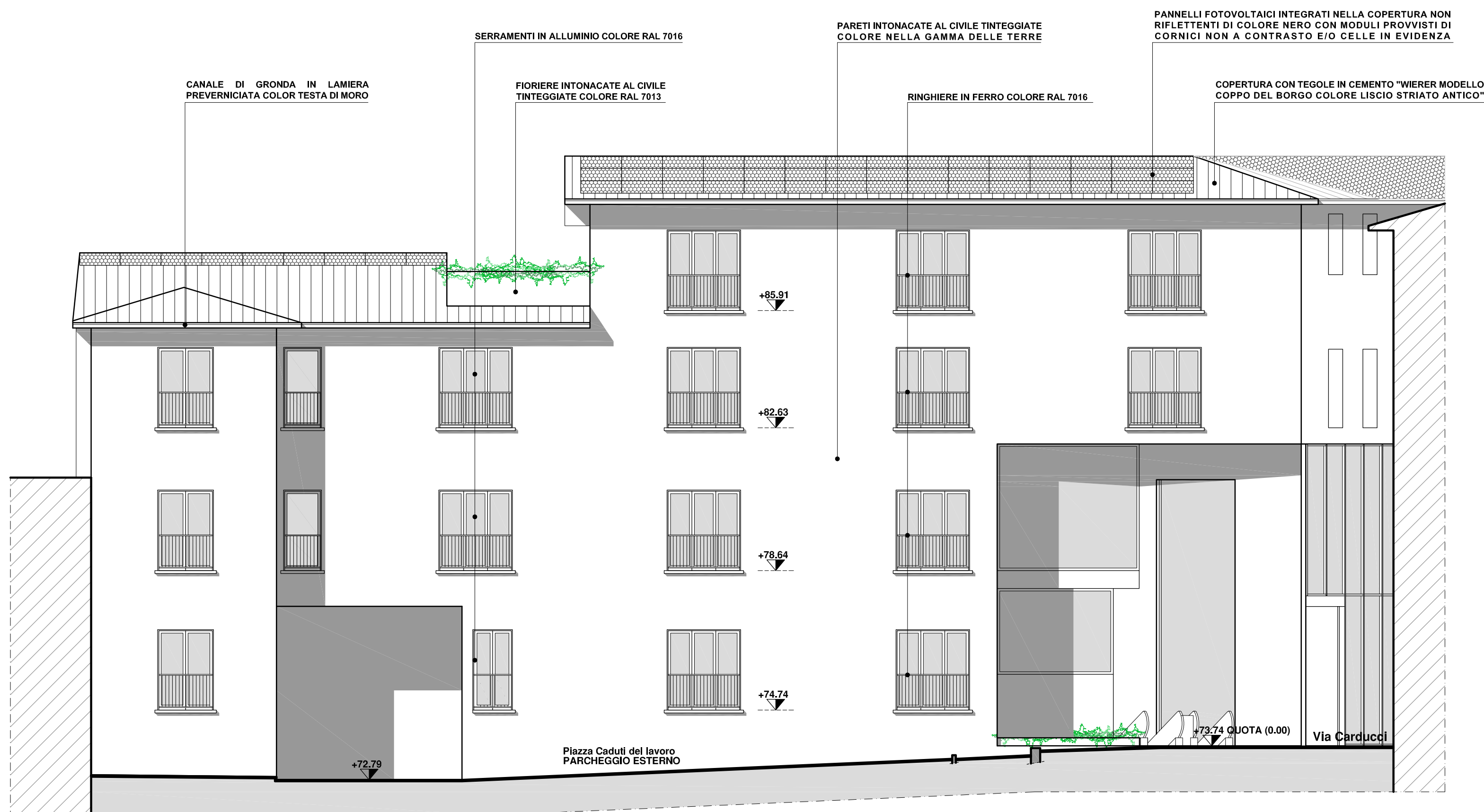
PROSPETTO NORD - VISTA DA PIAZZA CADUTI
