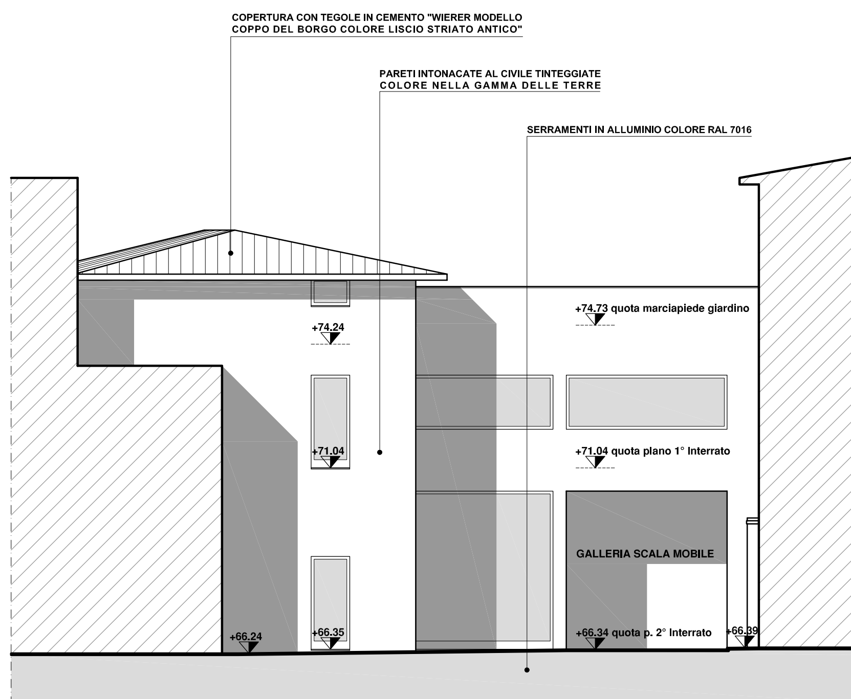
PROSPETTO EST - VISTA DA GALLERIA COMMERCIALE
