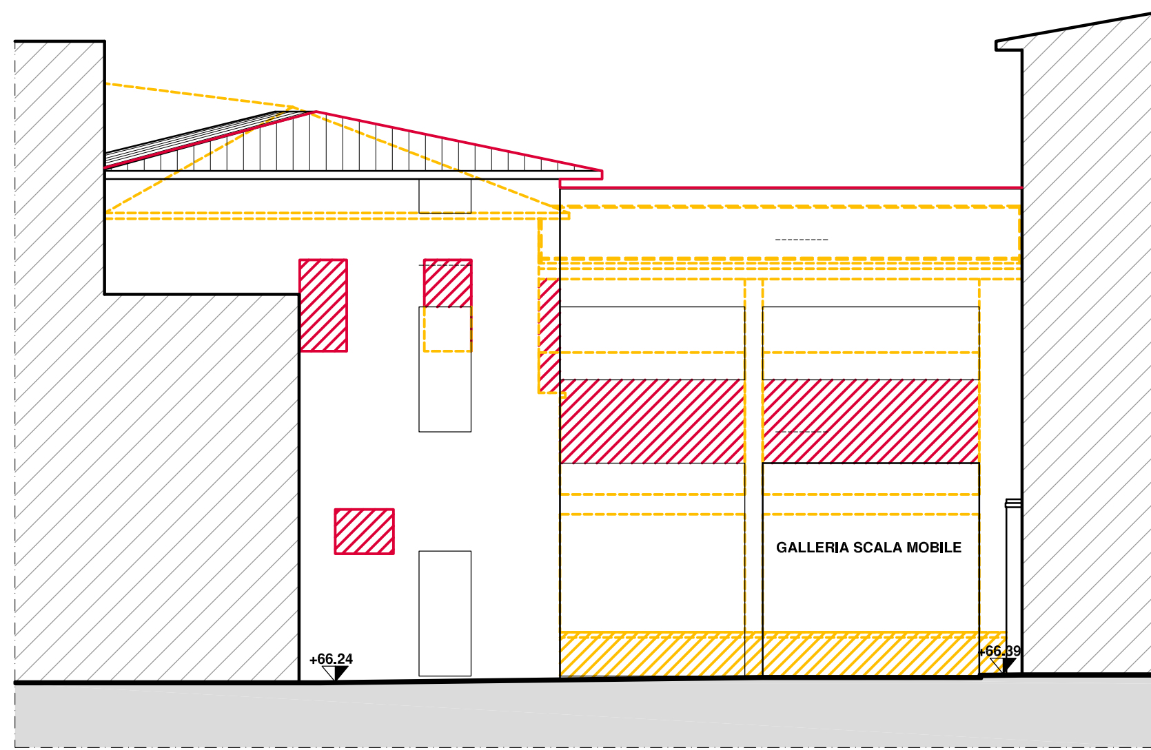
PROSPETTO EST - VISTA DA GALLERIA COMMERCIALE
